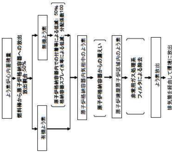
図 4.2 原子炉冷却材喪失の放射性核種の放出経路 (BWR 型原子炉施設)
