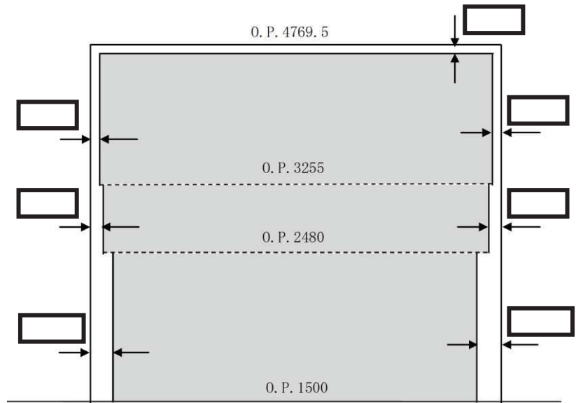
B-B' 断面図
