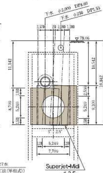
B-B断面図
