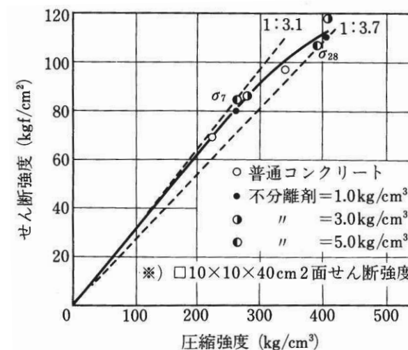
圧縮強度とせん断強度の関係例 ※2
