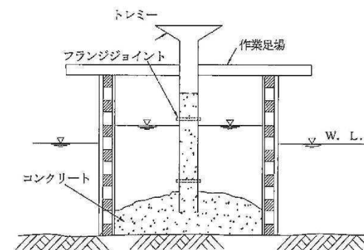
解説 図 8.2.1 トレミーによる水中コンクリートの打込み例
