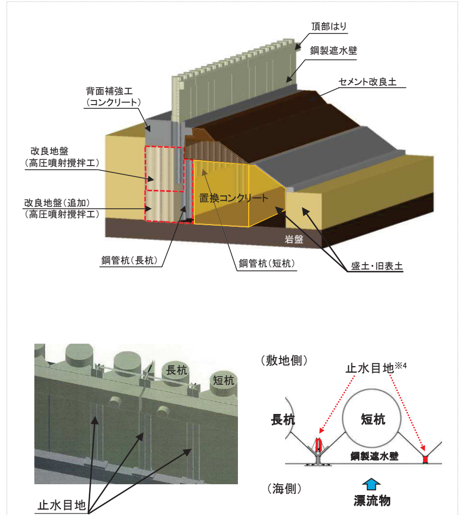
女川原子力発電所 鋼管式鉛直壁(一般部)
