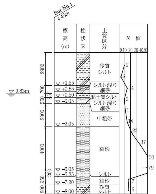
柱状図
