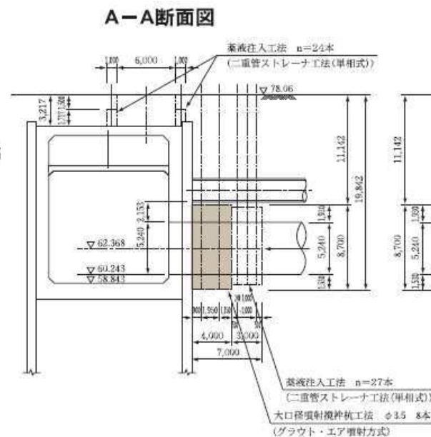
地盤改良概要図
