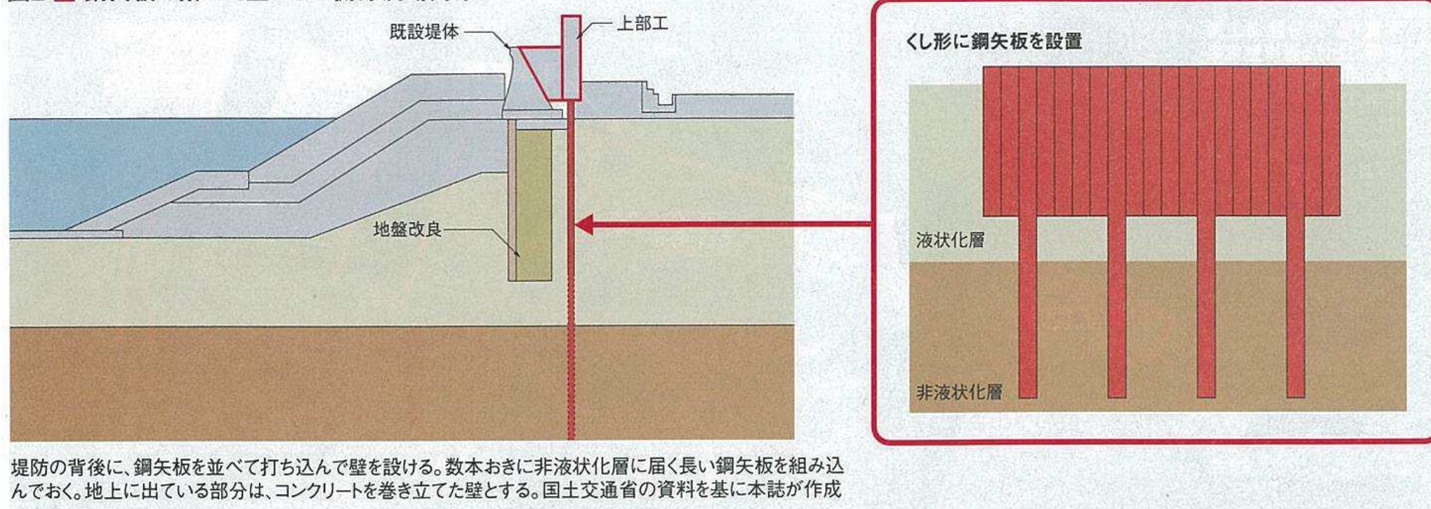
図2 ■ 鋼矢板で築いた壁による側方流動対策
