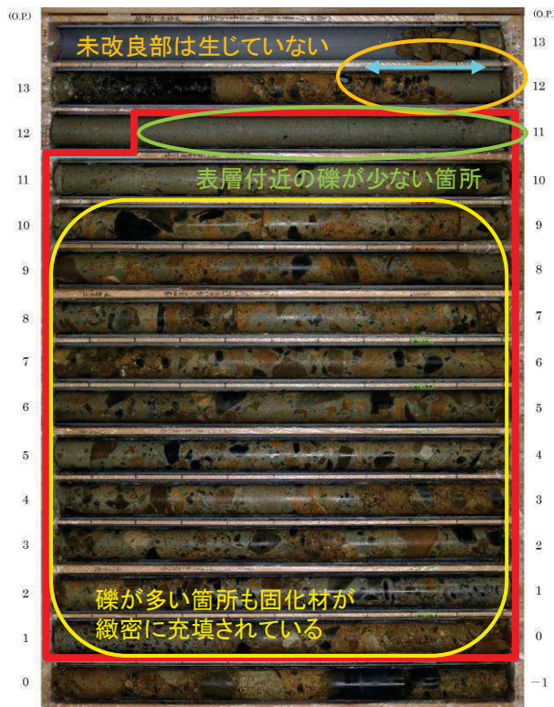
①孔 ボーリングコア写真
