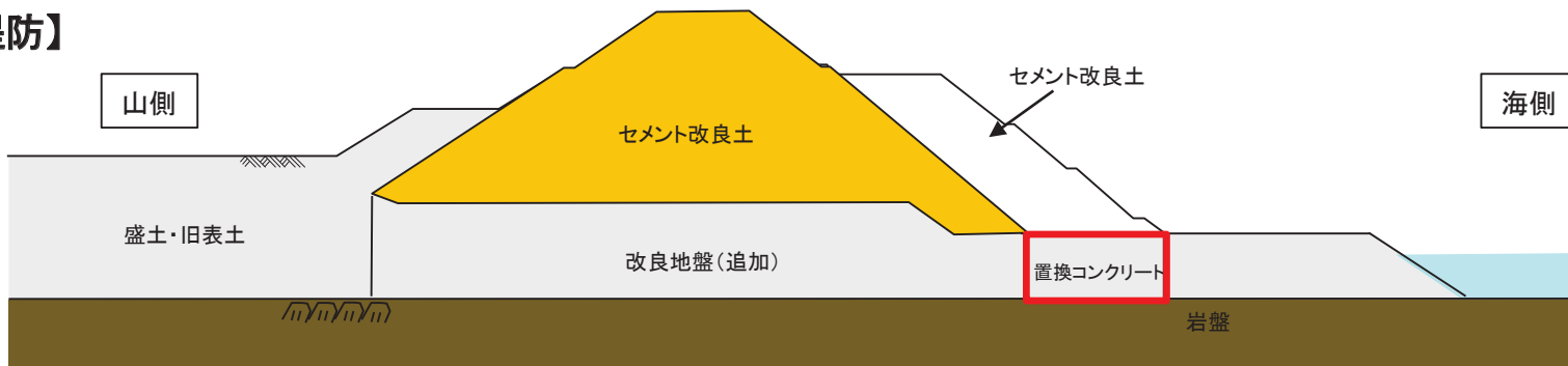
置換コンクリートの施工範囲
