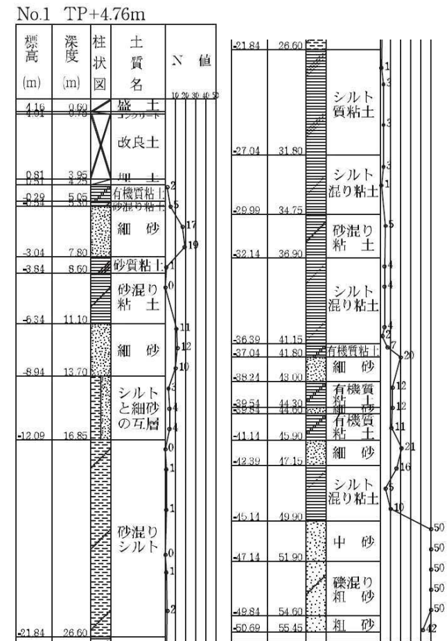
柱状図
