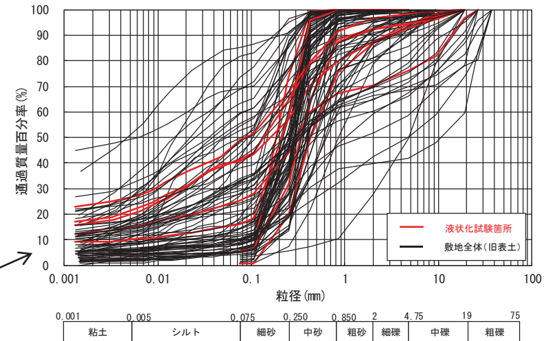
粒度分布
