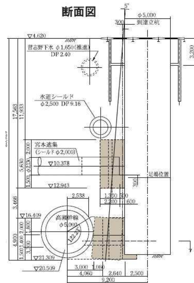
地盤改良概要図
