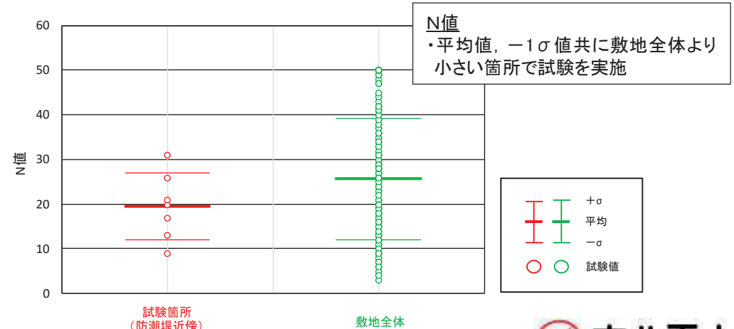
N値
