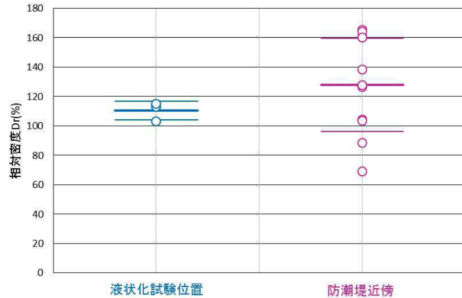
相対密度
