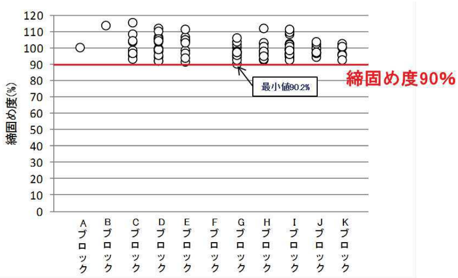
締固め度(各ブロック)
