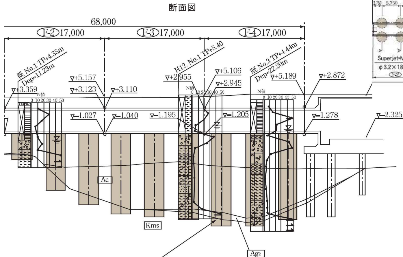
地盤改良概要図
