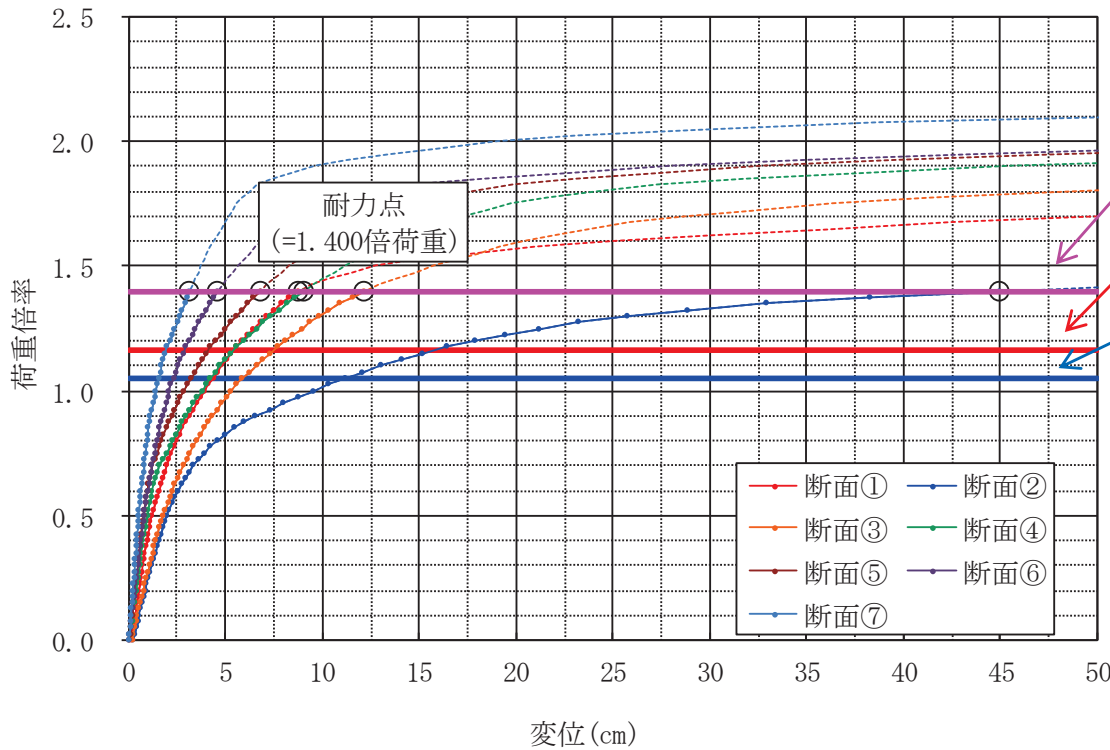
荷重倍率—変位関係
