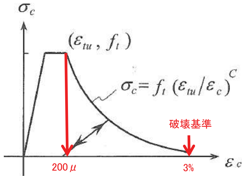
図 コンクリートの引張領域での平均応力-平均ひずみ関係の例 (コンクリート標準示方書2017)
