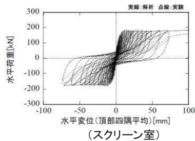
図 水平変位－水平荷重関係
