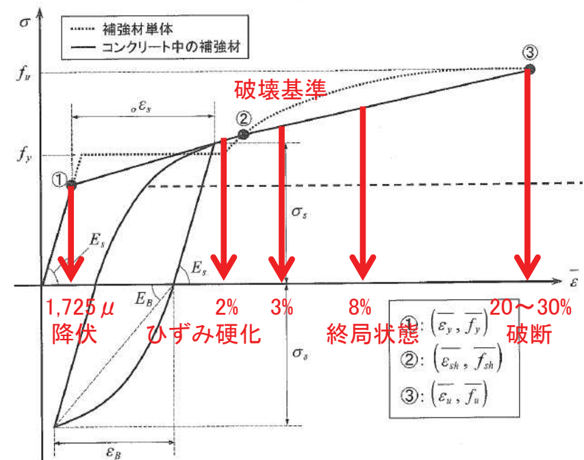
図 鉄筋の履歴モデル (コンクリート標準示方書2017)
