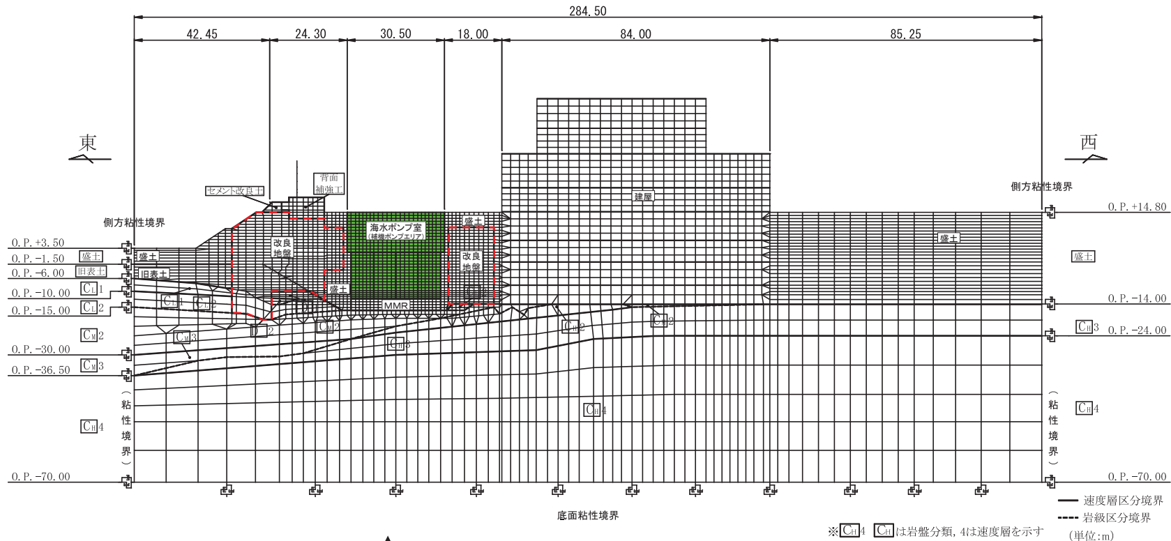
二次元地震応答解析(解析モデル図:補機ポンプエリア)
