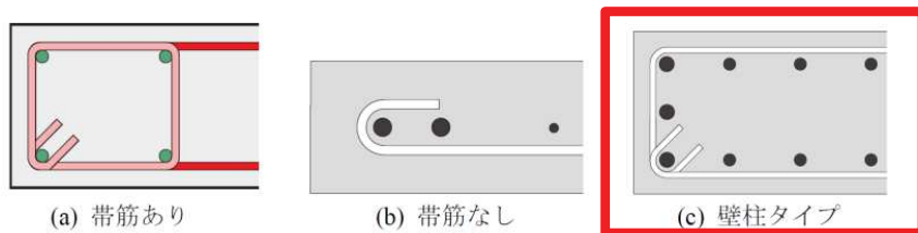
図 無開口・矩形断面の分類 ※2
