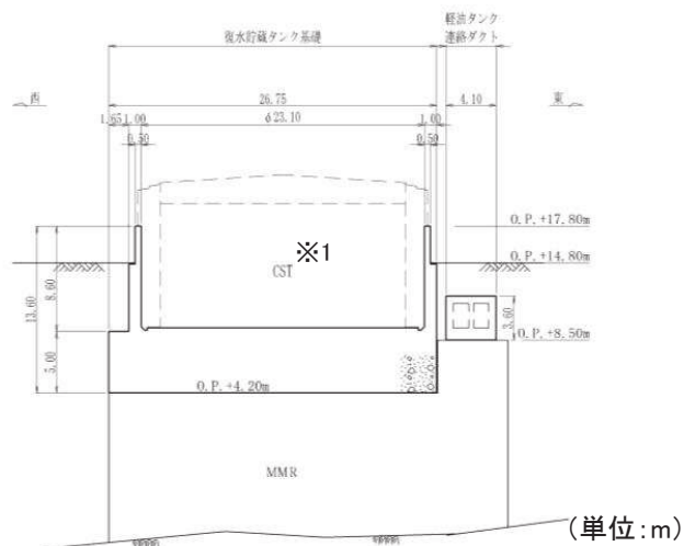
復水貯蔵タンク基礎断面図(B-B断面)
