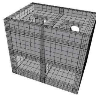
(c) ポンプ室
