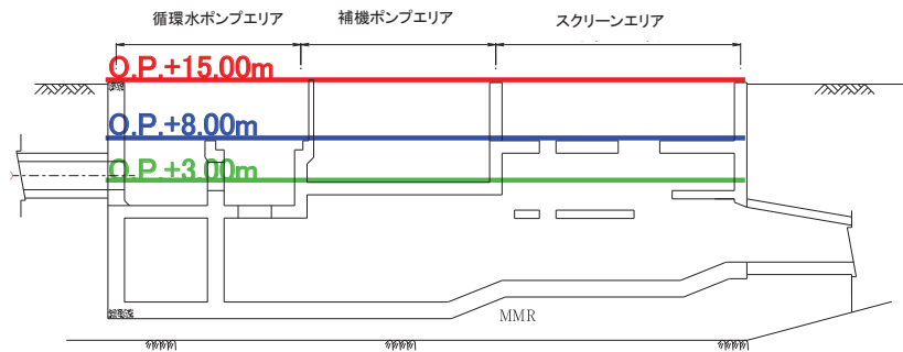
縦断面図
