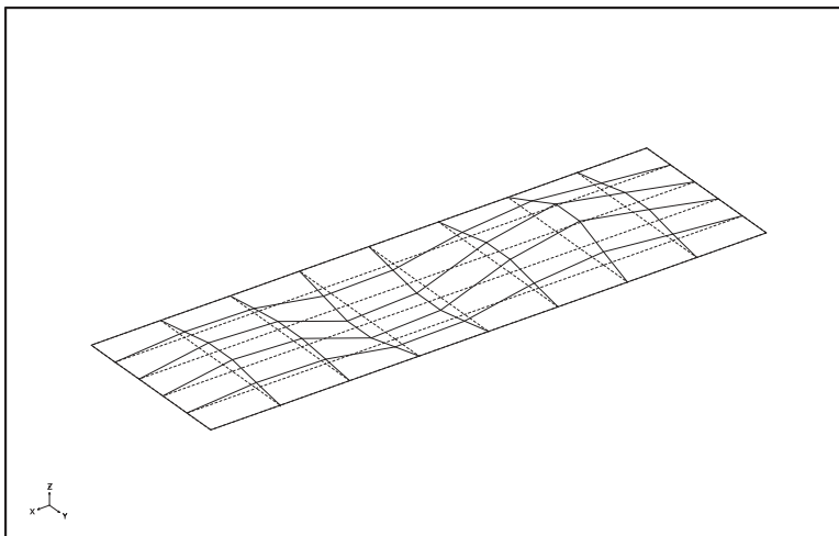
3次モード
