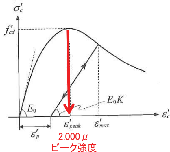
図 簡略化したコンクリートの圧縮領域の履歴モデル (コンクリート標準示方書2017)
