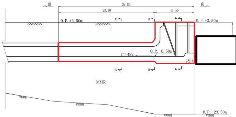
取水口縦断面図
