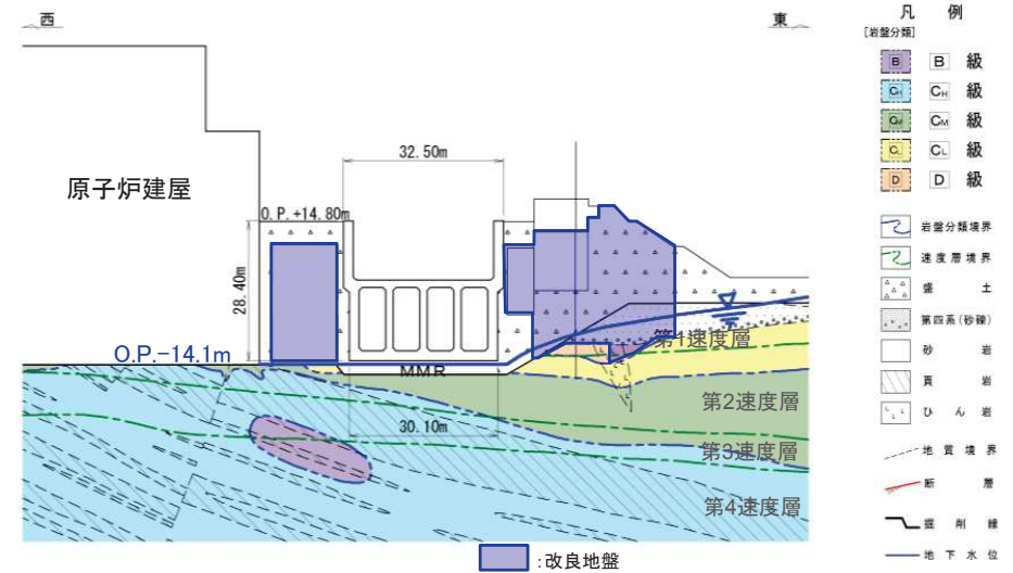
改良範囲断面図(A-A' 断面)
