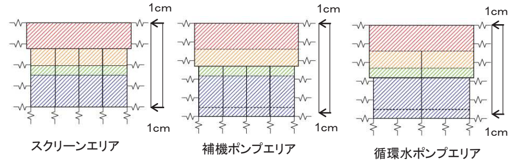
二次元等価剛性モデル
