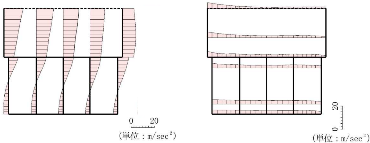
応答加速度分布(例)
