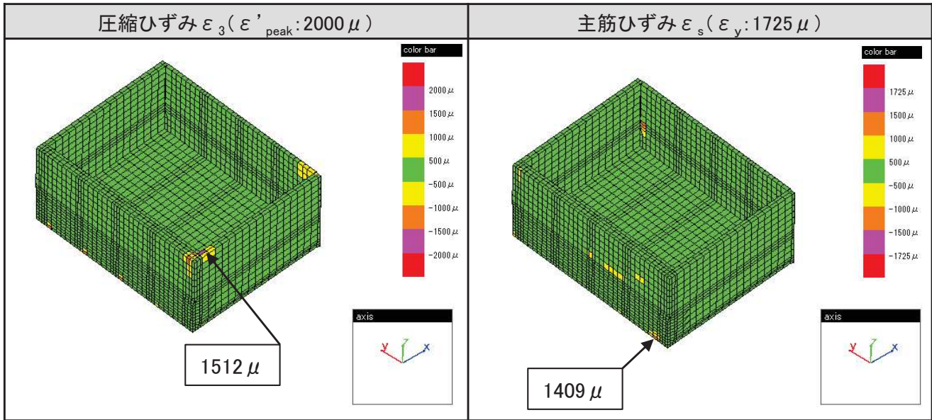
抽出位置(精査中)
