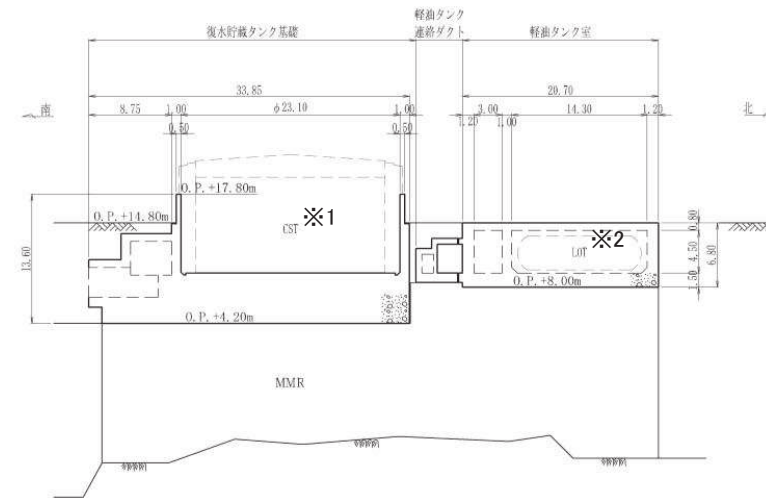
軽油タンク室・復水貯蔵タンク基礎 断面図(A-A断面)
