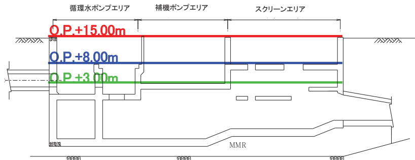
縦断面図
