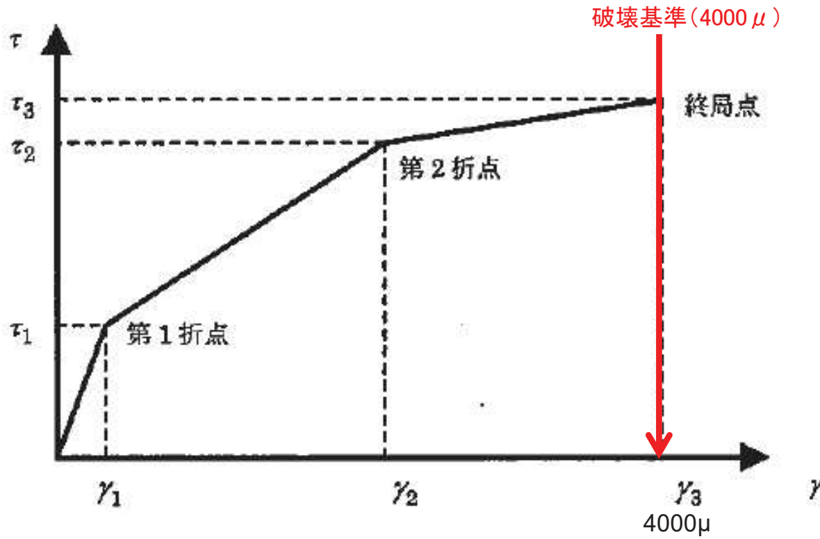
トリリニア・スケルトンカーブ
