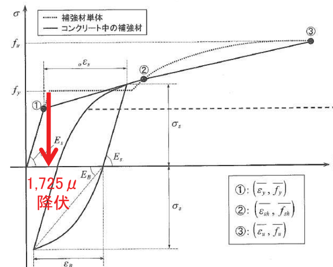
図 鉄筋の履歴モデル (コンクリート標準示方書2017)
