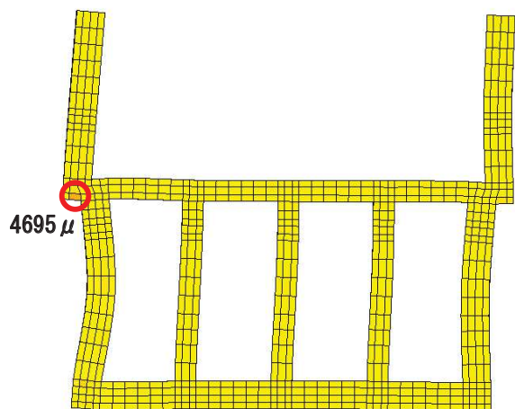
最大ひずみ発生箇所
