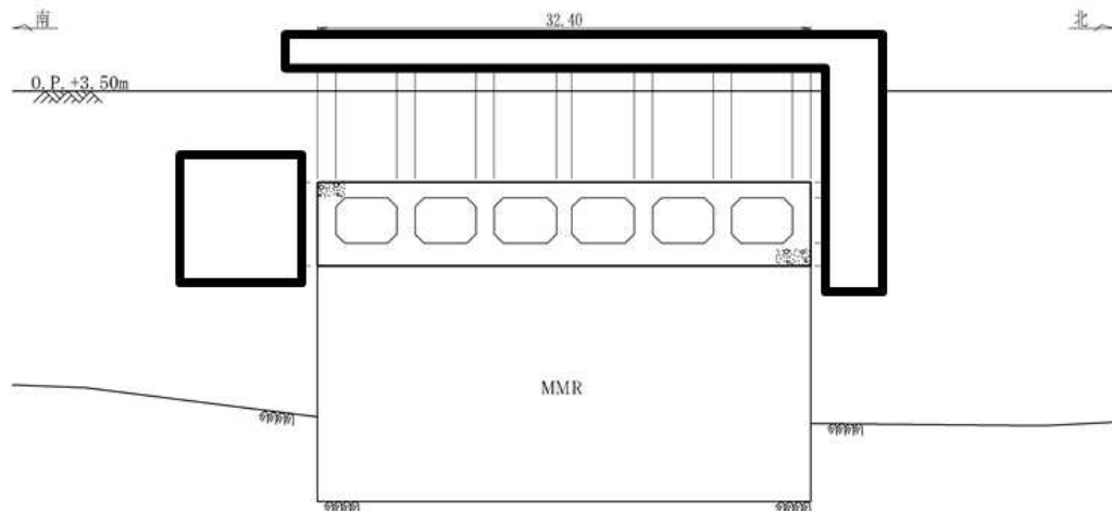
取水口(漸縮部)断面図(B-B断面)
