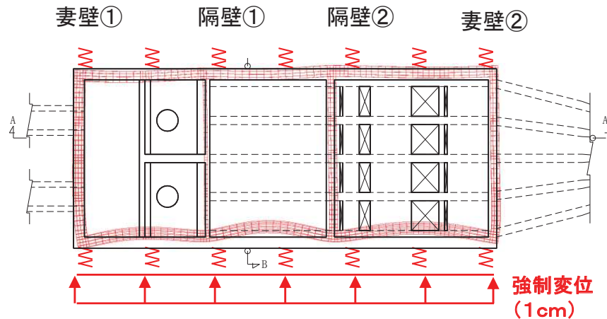
構造物天端 (O.P.+15.00m) の変形図
