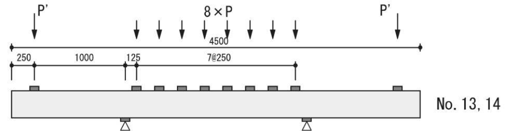
[ 立面図 ]
