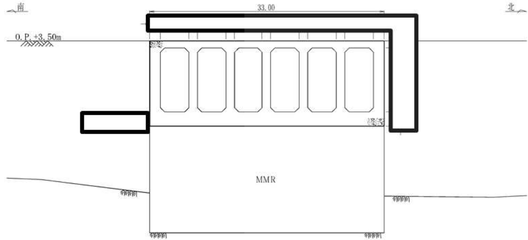
取水口(標準部)断面図(A-A断面)
