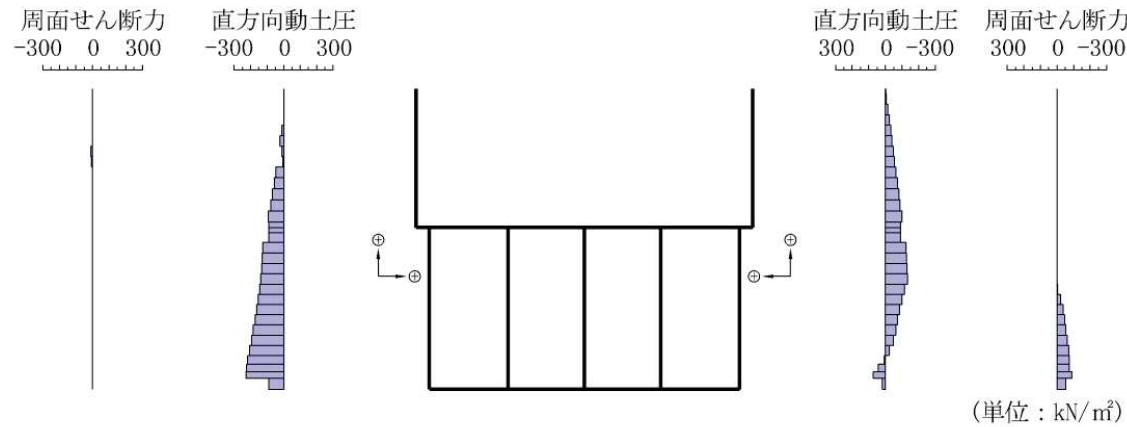
地震時増分土圧分布(例)
