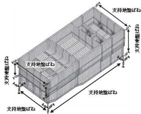
地震時解析
