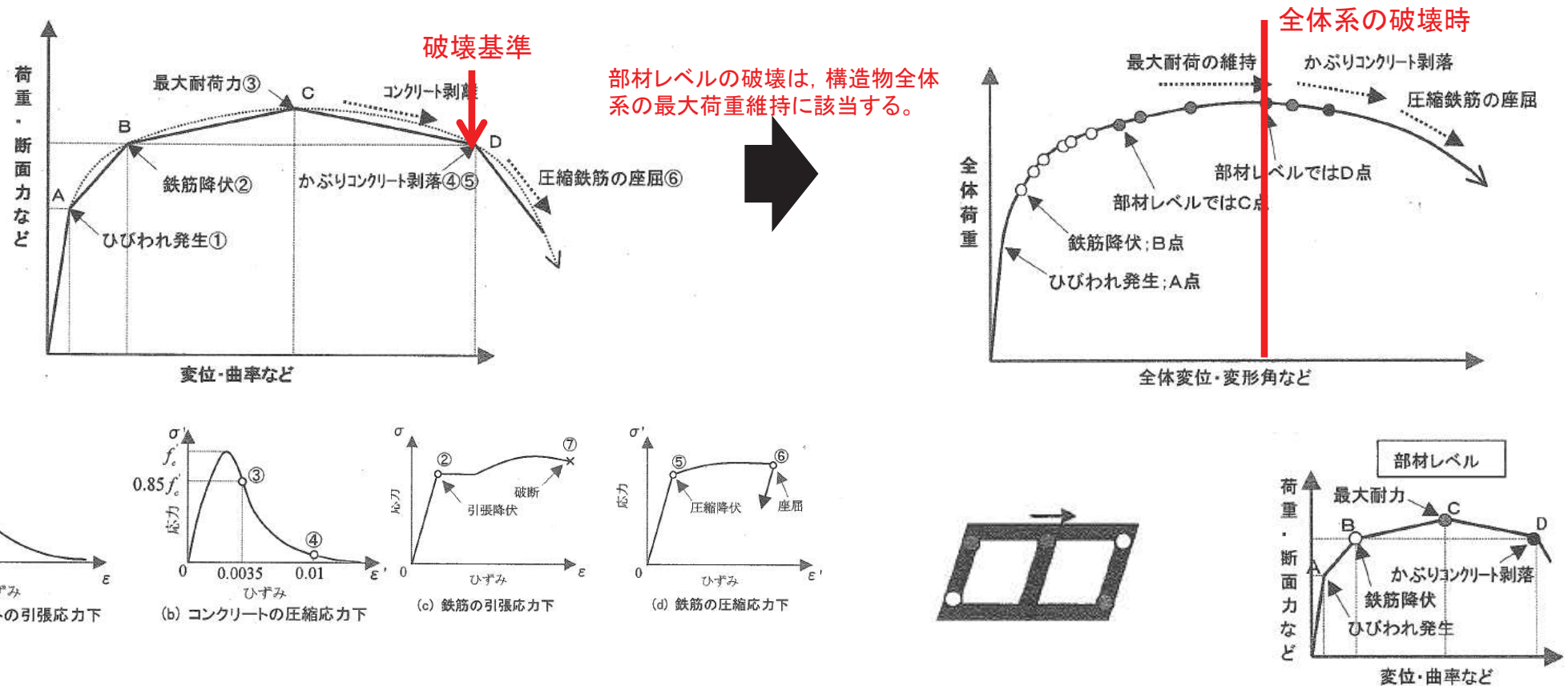
図 コンクリートと鉄筋の応力ひずみ関係に対する概念図 (原子力発電所屋外重要土木構造物の耐震性能照査指針<技術資料>) 図 構造物全体と部材レベルの損傷状態の対応関係に対する概念図 (原子力発電所屋外重要土木構造物の耐震性能照査指針<技術資料>)
