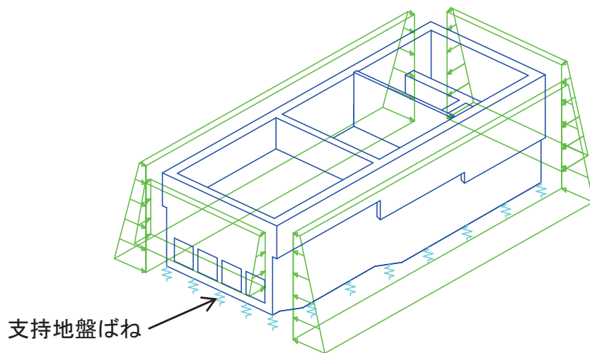
静止土圧載荷イメージ図
