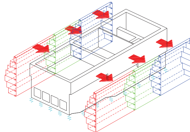
地震時荷重の分布形状イメージ
