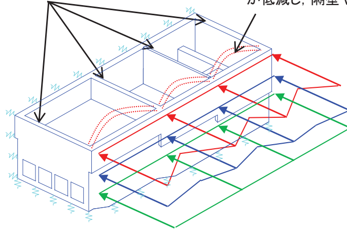
部材の変形を考慮した土圧分布イメージ
