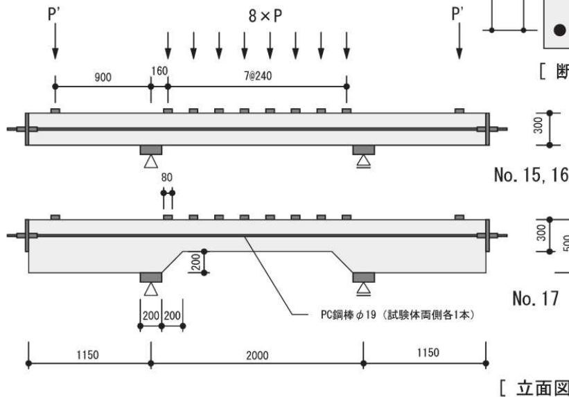
解析ケース15~17
