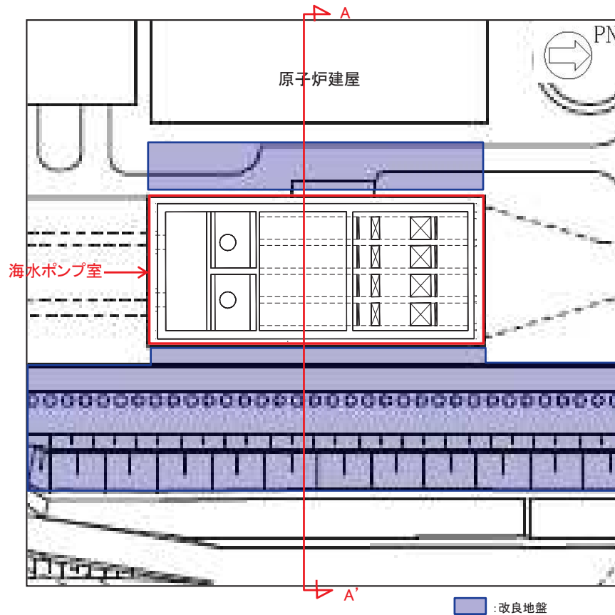
改良範囲平面図
