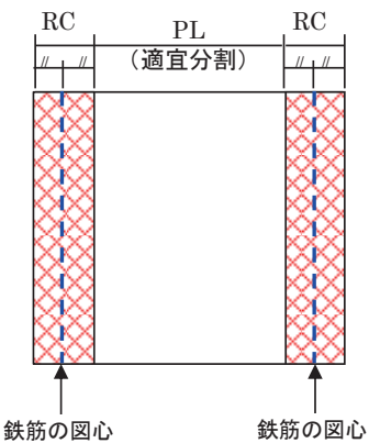
図 部材厚方向分割の概略図
