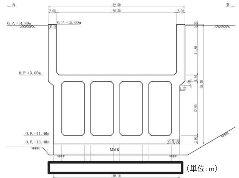
海水ポンプ室断面図(B-B断面)
