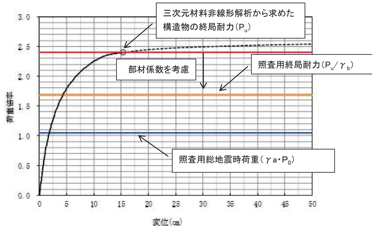
変位－荷重倍率関係図のイメージ
