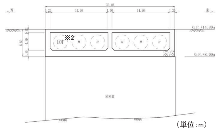
軽油タンク室断面図(C-C断面)
