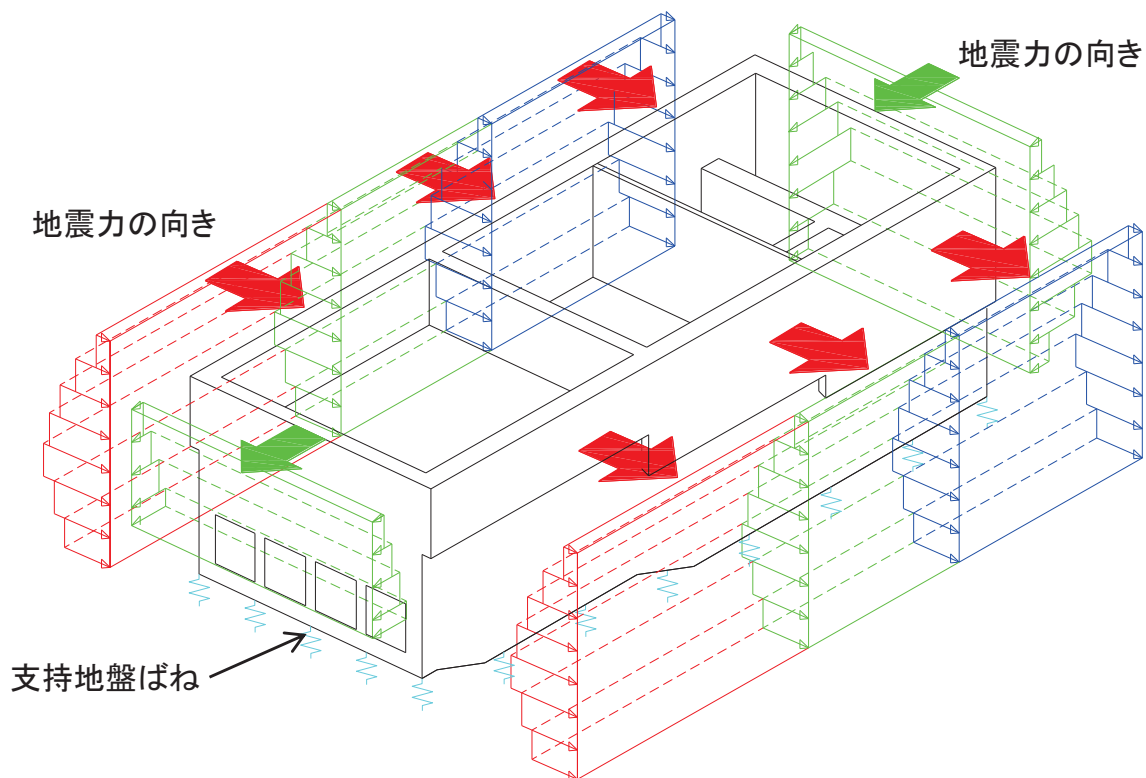
地震時荷重(2方向)載荷イメージ
