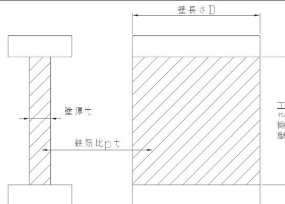
図 基本モデル(イメージ)
