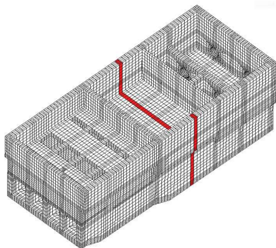
照査断面位置
