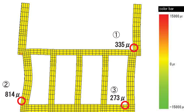
照査位置①～③
