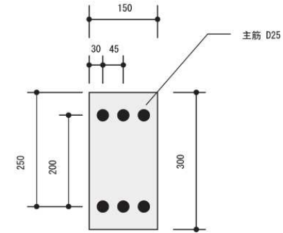
[ 断面図 ]
