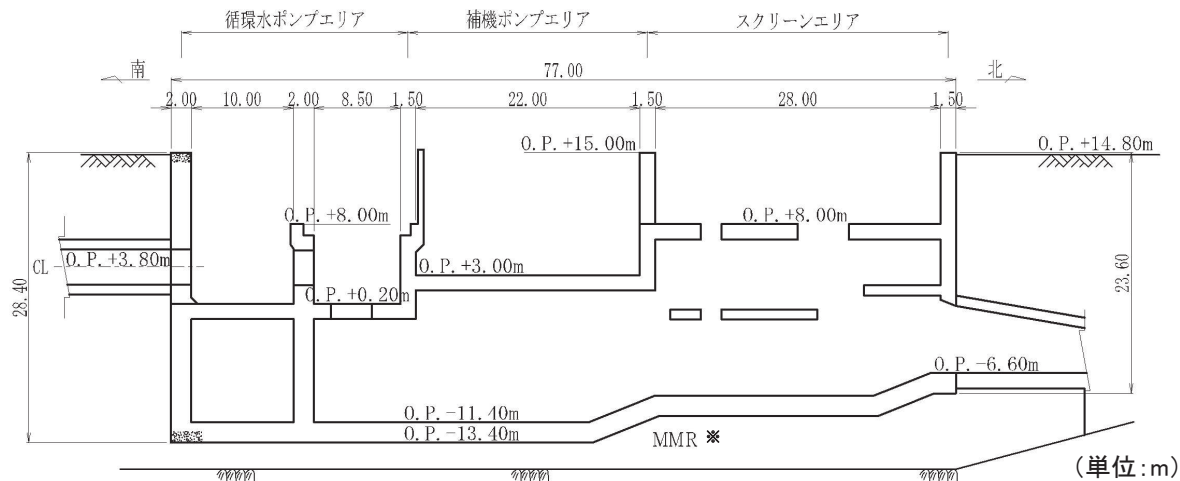
海水ポンプ室断面図(A-A断面)
