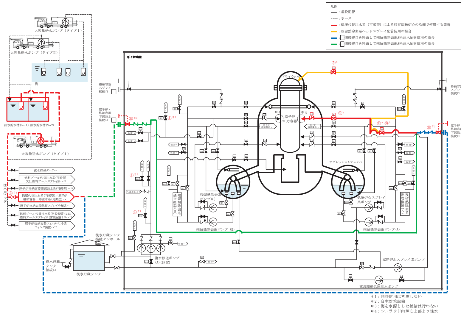
第 1.4.19 図 低圧代替注水系（可搬型）による残存溶融炉心の冷却 概要図（1/2）
