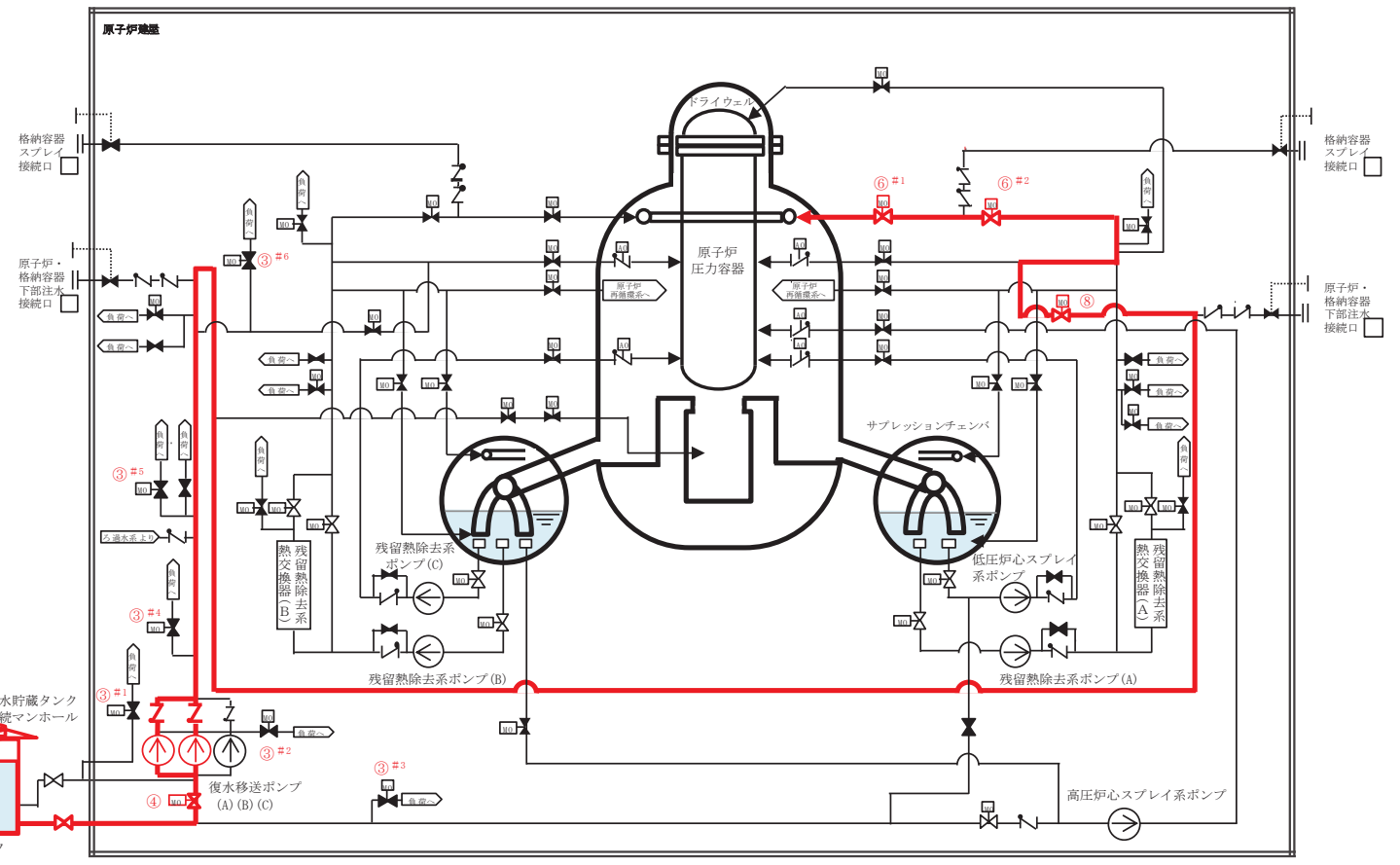
第 1.6.10 図 復水移送ポンプによるドライウエル内へのスプレイ 概要図 (1/2)
