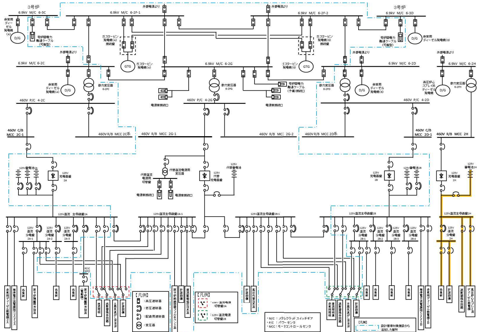
第 1.14.37 図 高圧炉心スプレイ系用直流電源設備による給電 概要図
