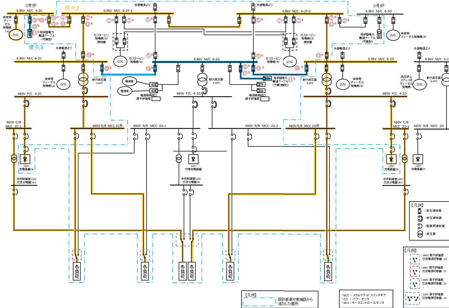
第 1.14.9 図 3号炉間電力融通ケーブルを使用した3号炉非常用ディーゼル発電機(A)系によるM/C2C系又はM/C2D系受電概要図
