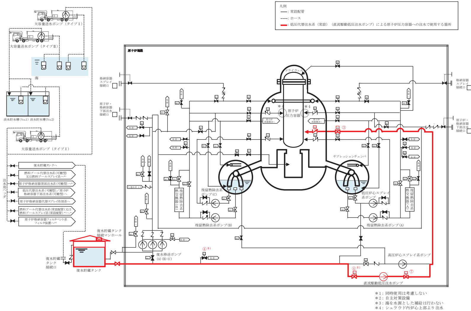
第 1.4.24 図 低圧代替注水系 (常設) (直流駆動低圧注水ポンプ) による原子炉圧力容器への注水 概要図 (1/2)
