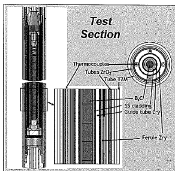
別図 2-6 BECHARRE 実験装置の概要とテストセクションの断
