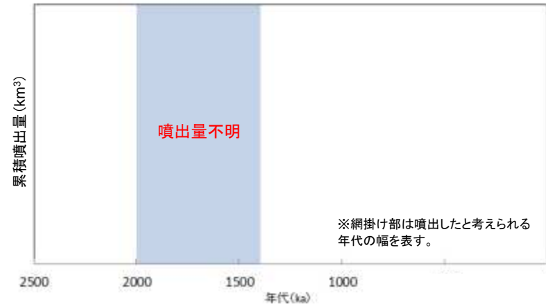
甑山の噴出量一年代階段ダイヤグラム
