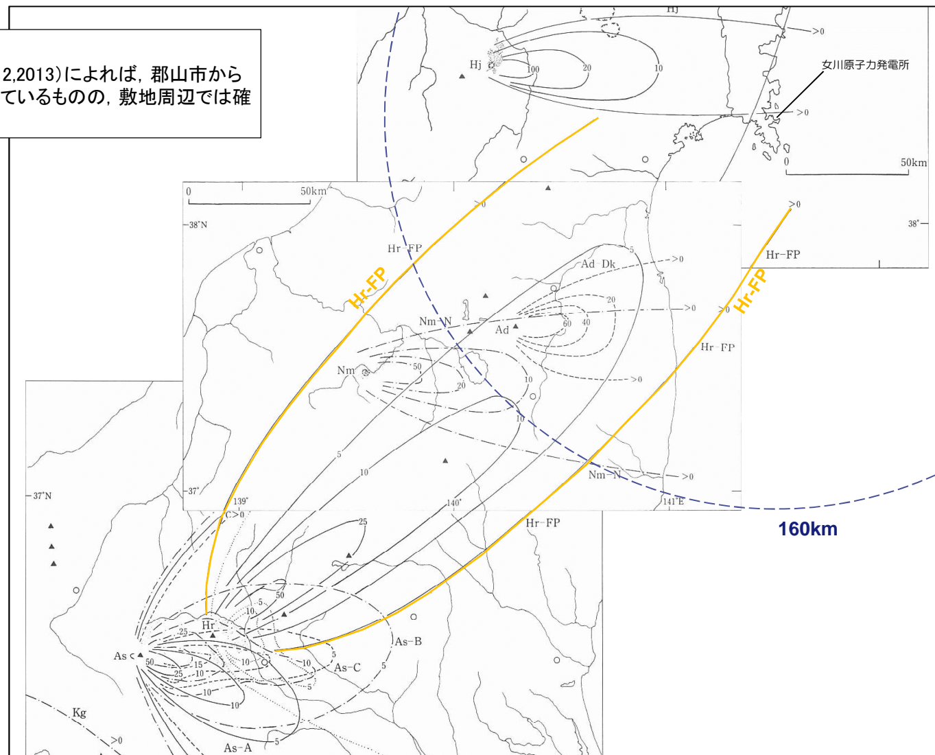
北関東～東北地方の主要テフラの等層厚線図 (町田・新井(2003)に一部加筆)
