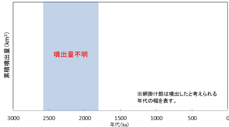
川尻三森山の噴出量-年代階段ダイヤグラム
