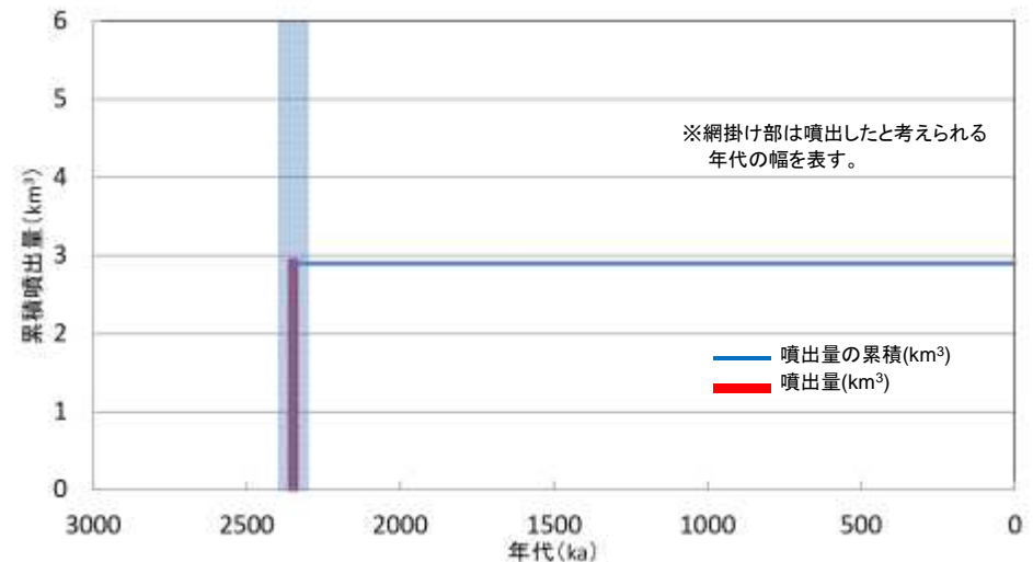
三吉葉山の噴出量一年代階段ダイアグラム
