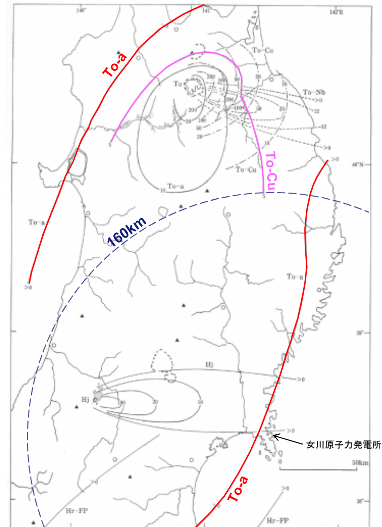
図3.4.2 東北地方の完新世主要テフラの等層厚線図 To-a 十和田a (pdfの分布も示す) [1][2][3] Hr-FP 榛名ニツ岳伊香保 [2] To-Cu 十和田中礫 [2] To-Nb 十和田南礫 [2] Hj 御折尾花沢 (pdfの分布も示す) [2] To: 十和田, Hj: 村松 [1] 宍倉ほか (2007a), [2] Araki et al. (1991), [3] Hayakawa (2005)
