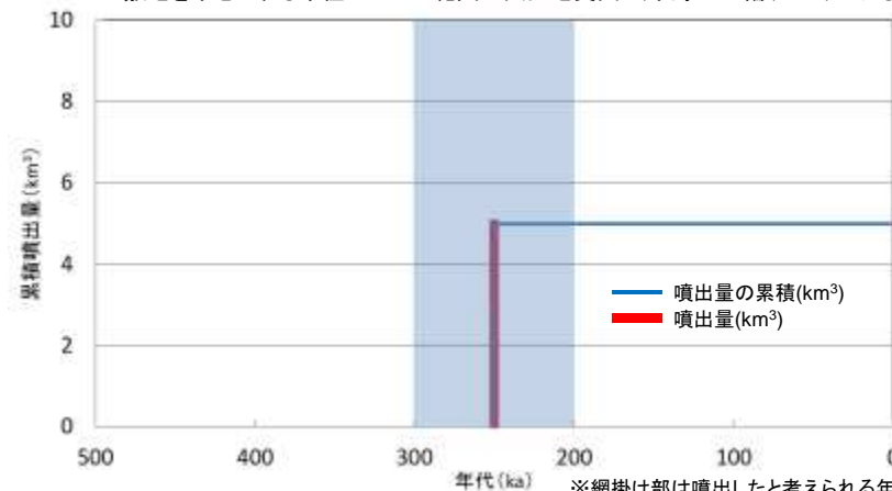
高松岳の噴出量-年代階段ダイヤグラム
