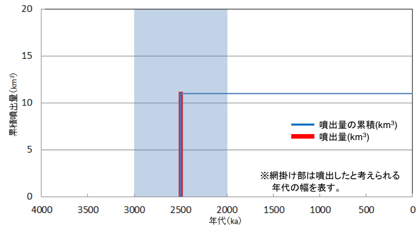
赤倉カルデラの噴出量－年代階段ダイヤグラム
