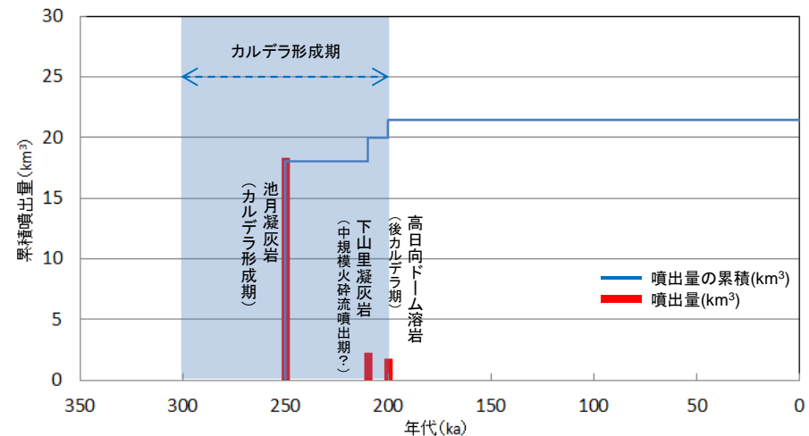
鬼首カルデラの噴出量-年代階段ダイアグラム
