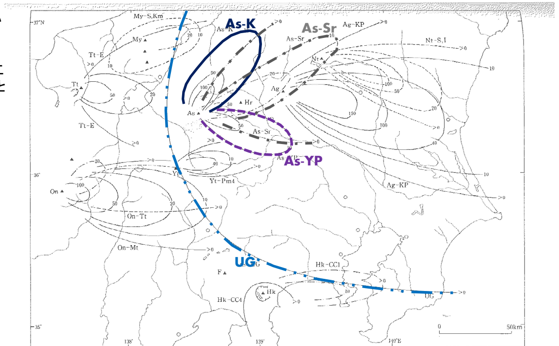
図 3.3-2 中部・関東地方の後期更新世主要テフラの等層厚線図(その1) Nt-S 男体七本塚 1) より編纂 Nt-I 男体今市 1) より編纂 UG 立川ローム上部ガラス質 2) など As-K 浅間草津 (pHの分布も示す) 3) As-YP 浅間板鼻黄色 (pHの分布も示す) 3) As-Sr 浅間白糸 3) Yt-Pm4 ハヶ岳 4),5) Ag-KP 赤城臨沼 6),7) My-S, Km 妙高四山・兼僕 7),8) Hk-CC4 箱根三島 9) Hk-CC1 箱根中央火口丘 1) Tt-E 立山E 2) より編纂 On-Mt 御岳三番 10) など On-Tt 御岳辰野 10) など Tt: 立山, My: 妙高, As: 浅間, Hr: 榛名, Ag: 赤城, Nt: 日光男体, On: 御嶽, Yt: ハヶ岳, F: 富士, Hk: 箱根, 1) 関東ローム研究グループ(1965), 2) 鈴木正幸(1991), 3) 中沢ほか(1984), 4) Kawachi et al.(1967), 5) 中谷(1970), 6) 鈴木毅(1990), 7) 早津・新井(1980), 8) 町田(1971), 9) 町田(1992), 10) 竹本ほか(1987)
