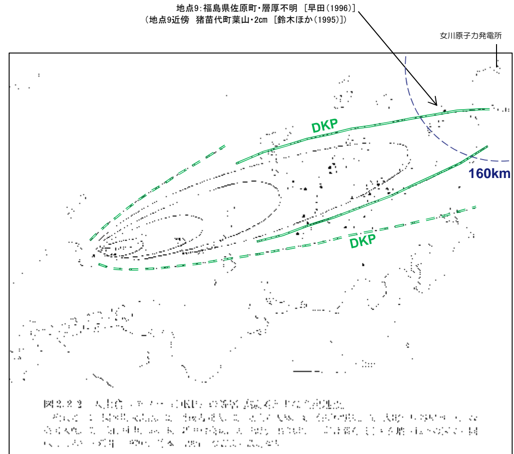
大山倉吉テフラの等層厚線図 (町田・新井(2003)に一部加筆)
