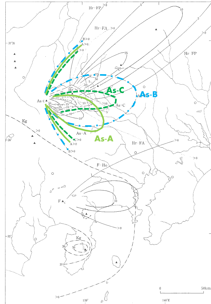
図 3.3-1 中部・関東地方の完新世主要テフラの等層厚線図
