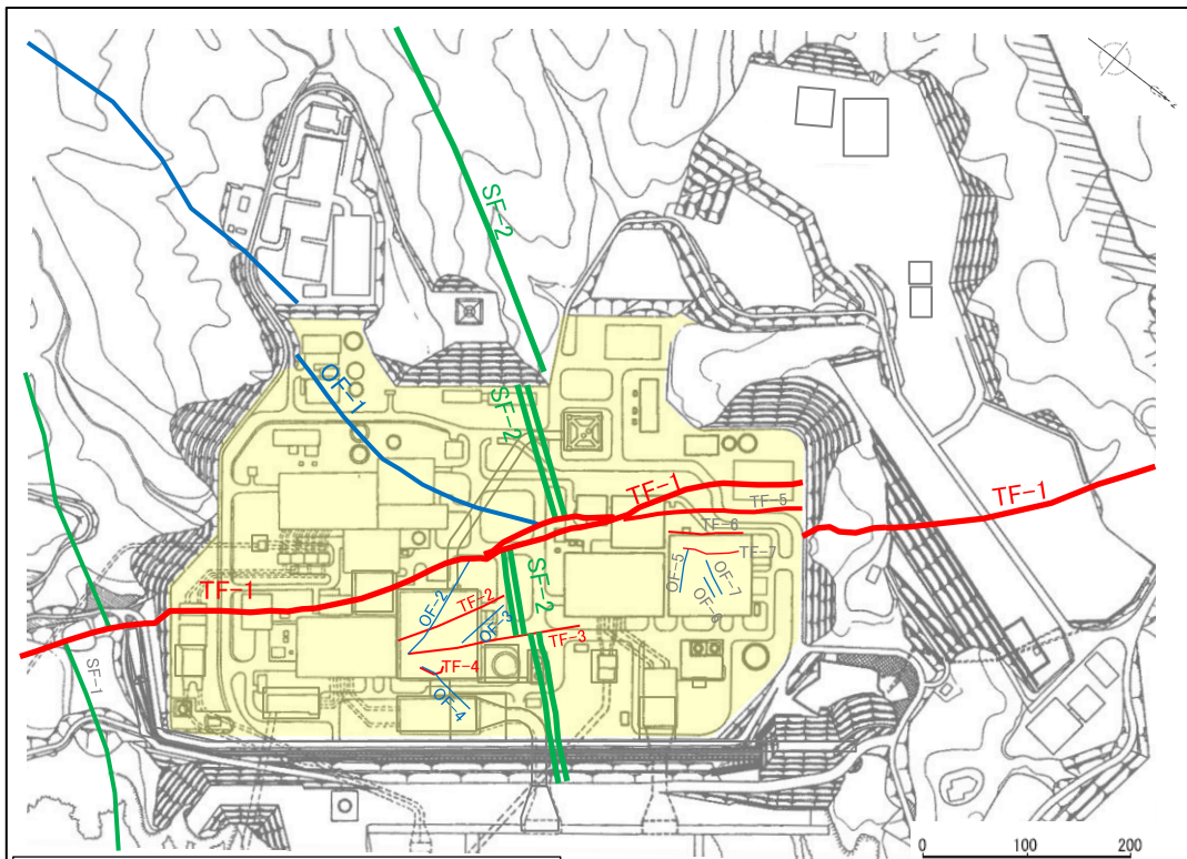
※黄色のハッチング箇所はO.P.約14mでの断層位置を示し、周囲は地質構造図による断層位置を示す。
