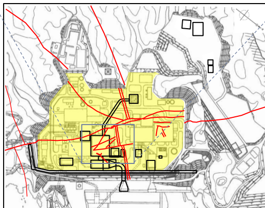
2号炉試掘坑と断層の位置関係
