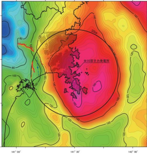
重力異常と地質構造
