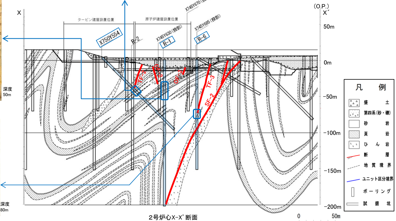
2号炉心X-X'断面
