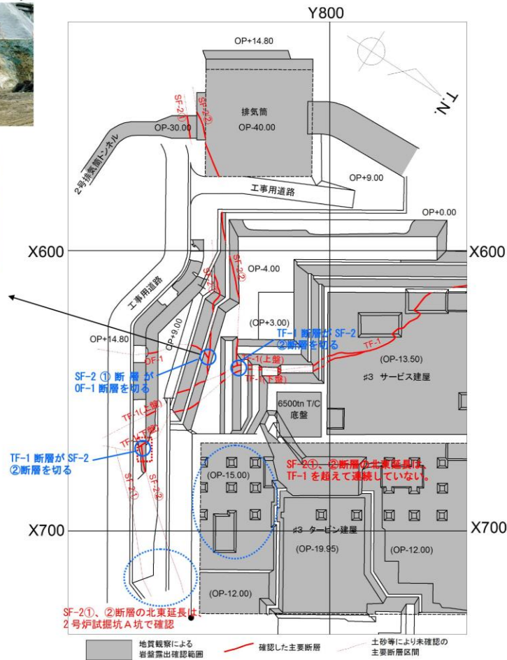
<3号炉関連の掘削面観察状況(抜粋)>
