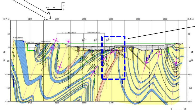
試掘坑内のSF-2①断層の延長位置 R-6孔深度98.50~98.20m (中石含む)
