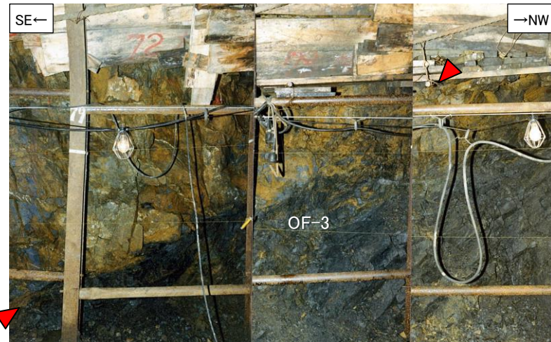
2号炉試掘坑A坑南西壁で確認したOF-3断層(左:写真, 右:スケッチ)
