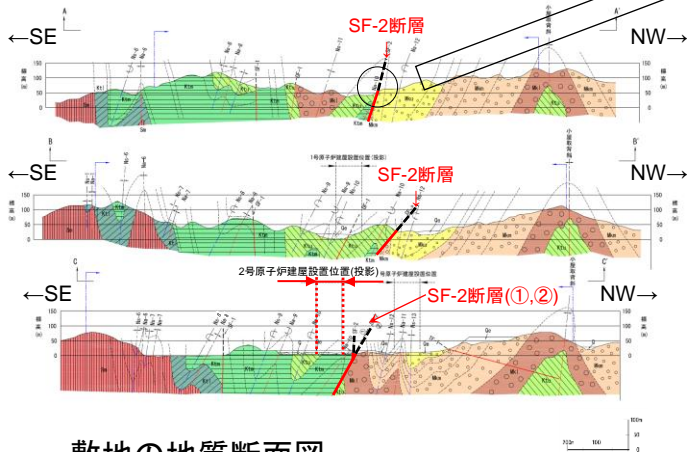
敷地の地質断面図
