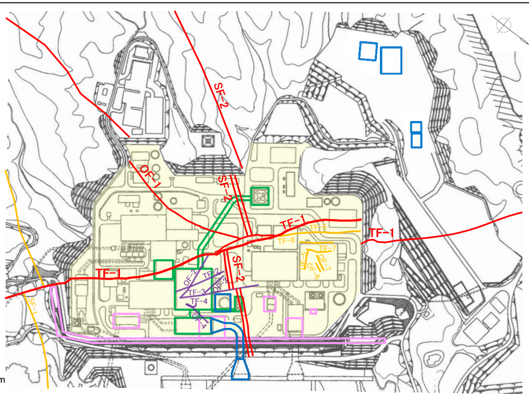
断層の切り切れ関係を示す模式図
