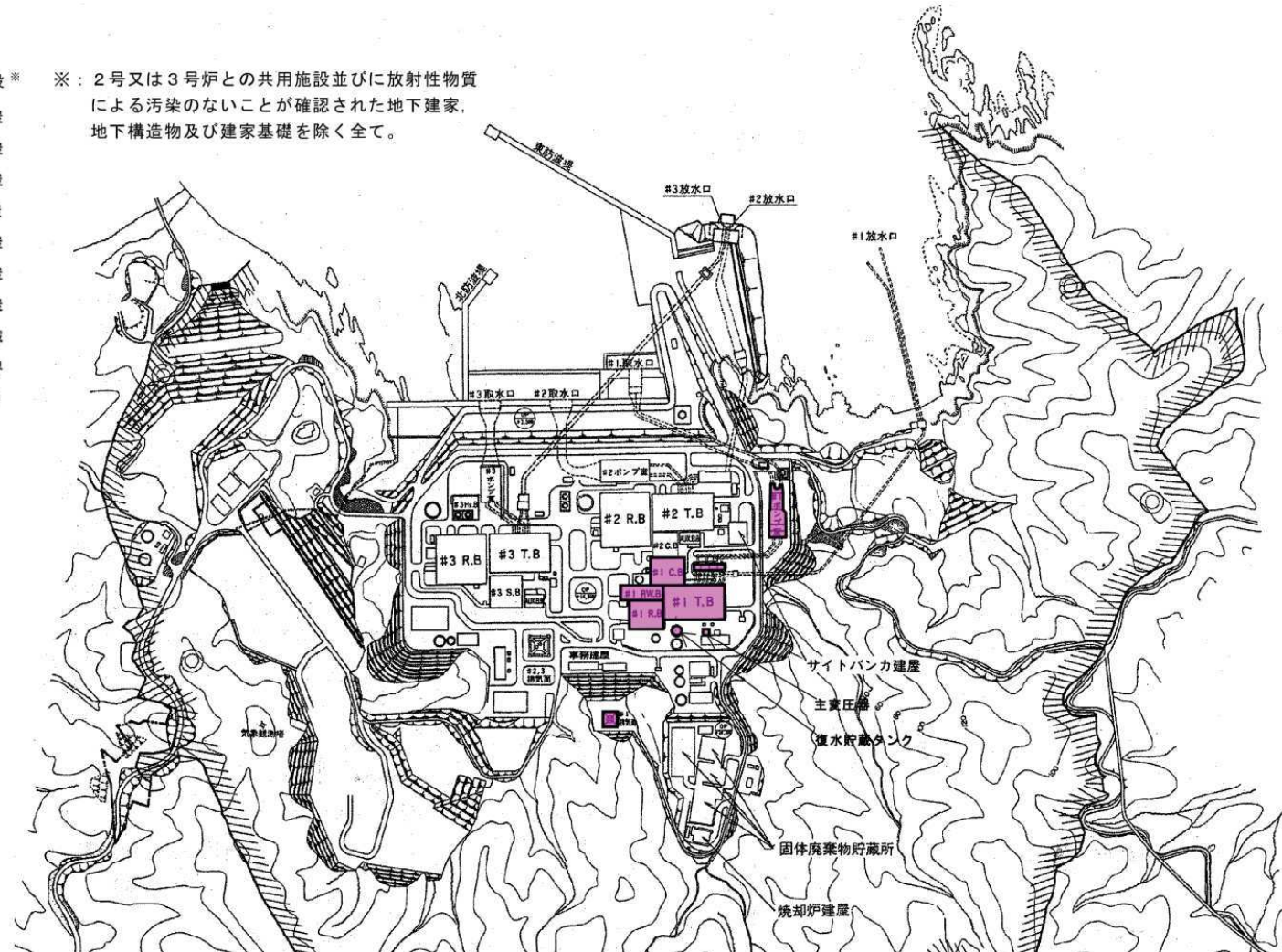
解体対象施設の配置図
