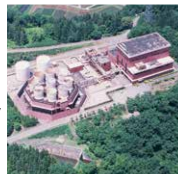
単機として国内最大の出力を誇る柳津西山地熱発電所(最大出力65,000kW)(福島県柳津町)
